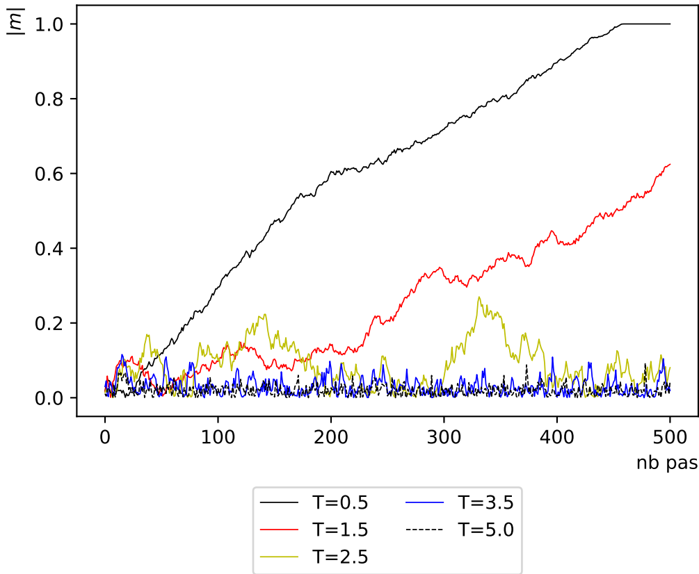
Evolution de l'aimantation sur 500 pas de Monte Carlo, N=64
